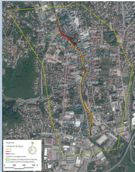
Carte 1: Système d'endiguement du Garon - Brignais (SE1)
