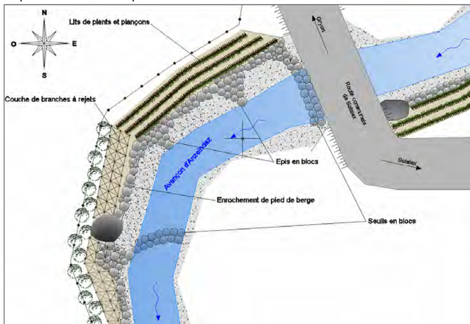
Fig. 2. Plan de situation.
