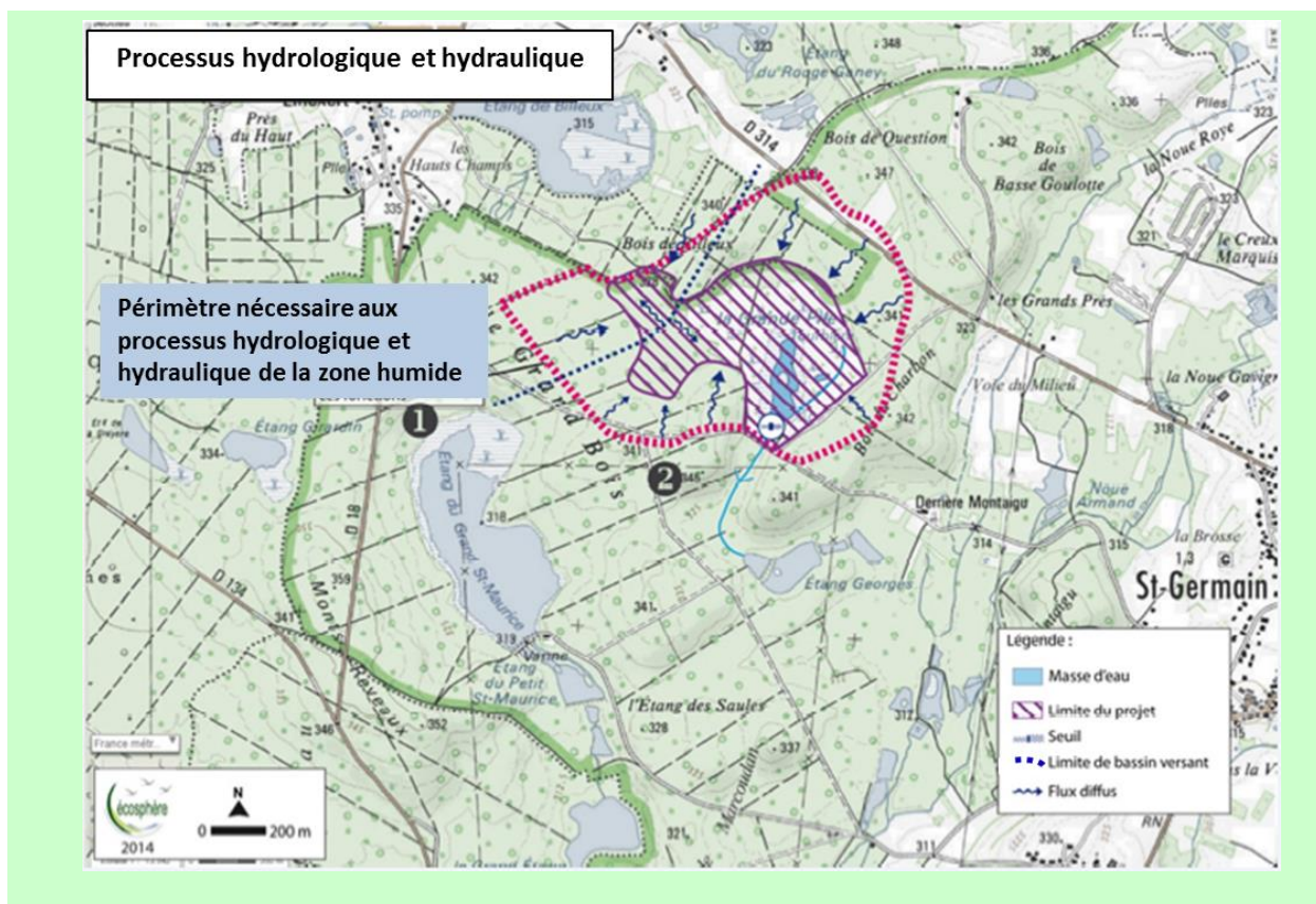
Figure 10 : exemple de délimitation du processus hydrologique et hydraulique (adaptée d'après les retours d'expérience des plans de gestion).
