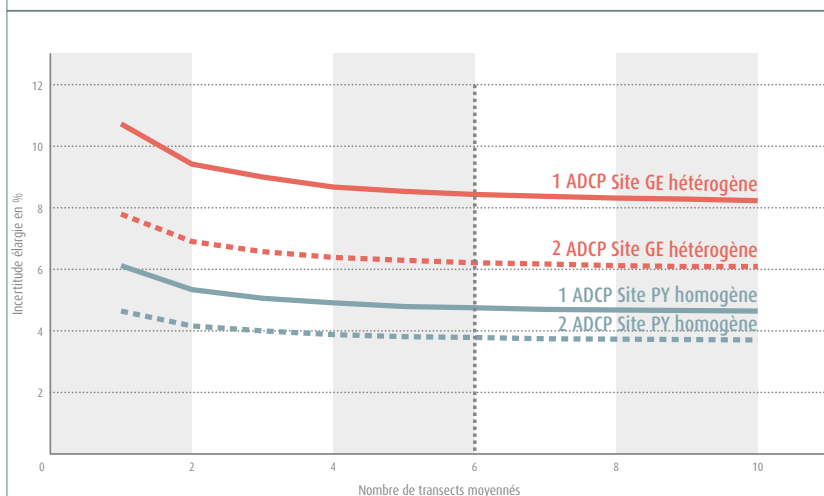
FIGURE 4.16 : RÉSULTAT D'INTERCOMPARAISONS POUR 2 SITES DU RHÔNE (LE COZ ET AL, 2016)
